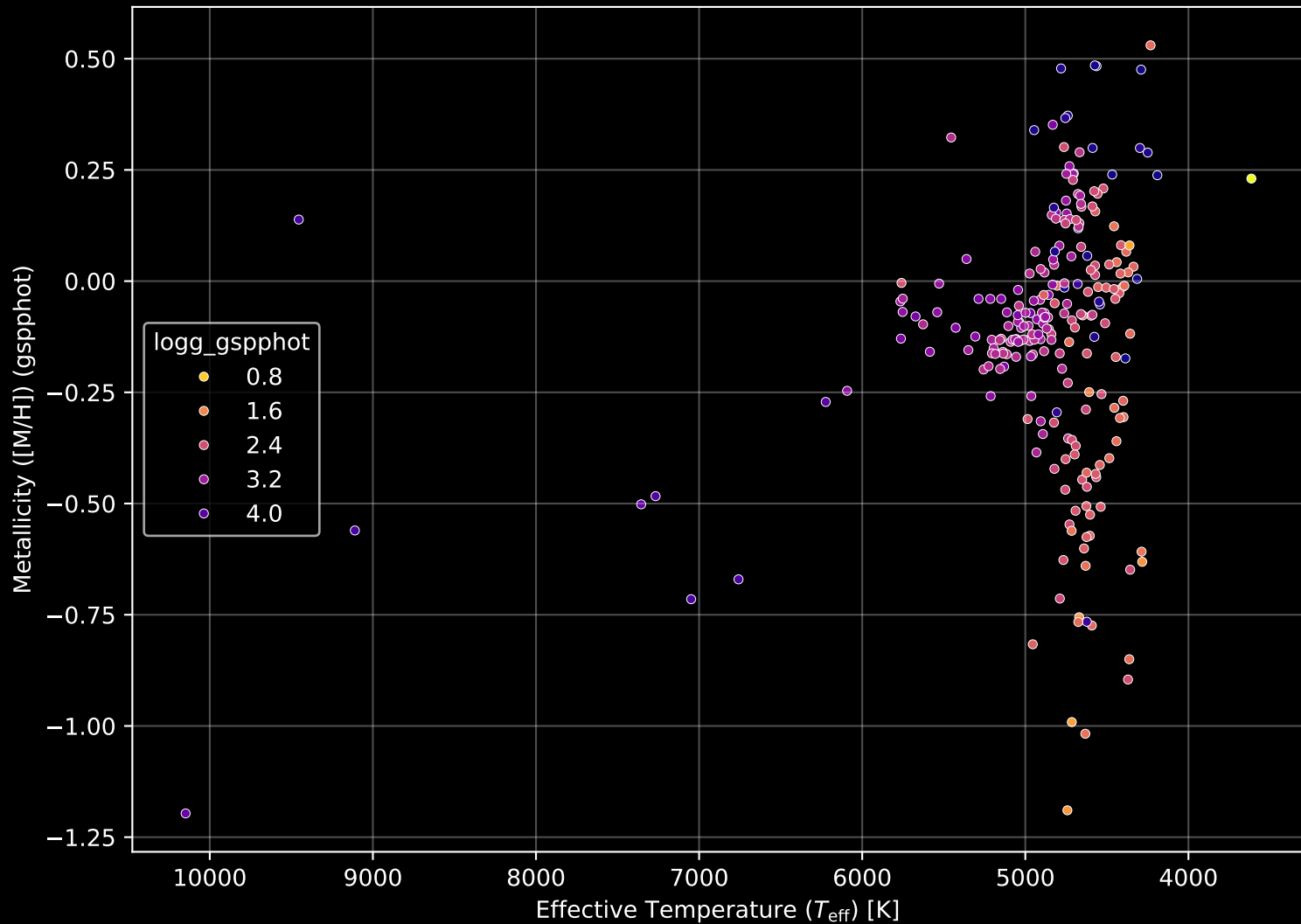
APOGEE DR17 Field: [296+12] Stellar Population Parameters (n= 243)
